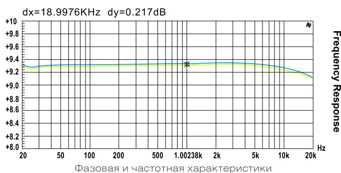
Фазовая и частотная характеристики
